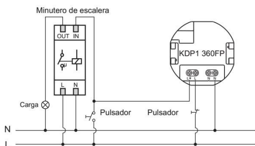
Control de minutero de escalera (El temporizador debe estar ajustado en la posición \sqrt{1s} .)
